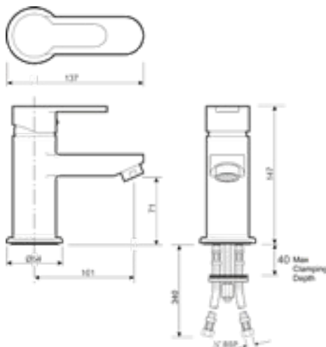
Mono Mixer Tap - SF5357CP
